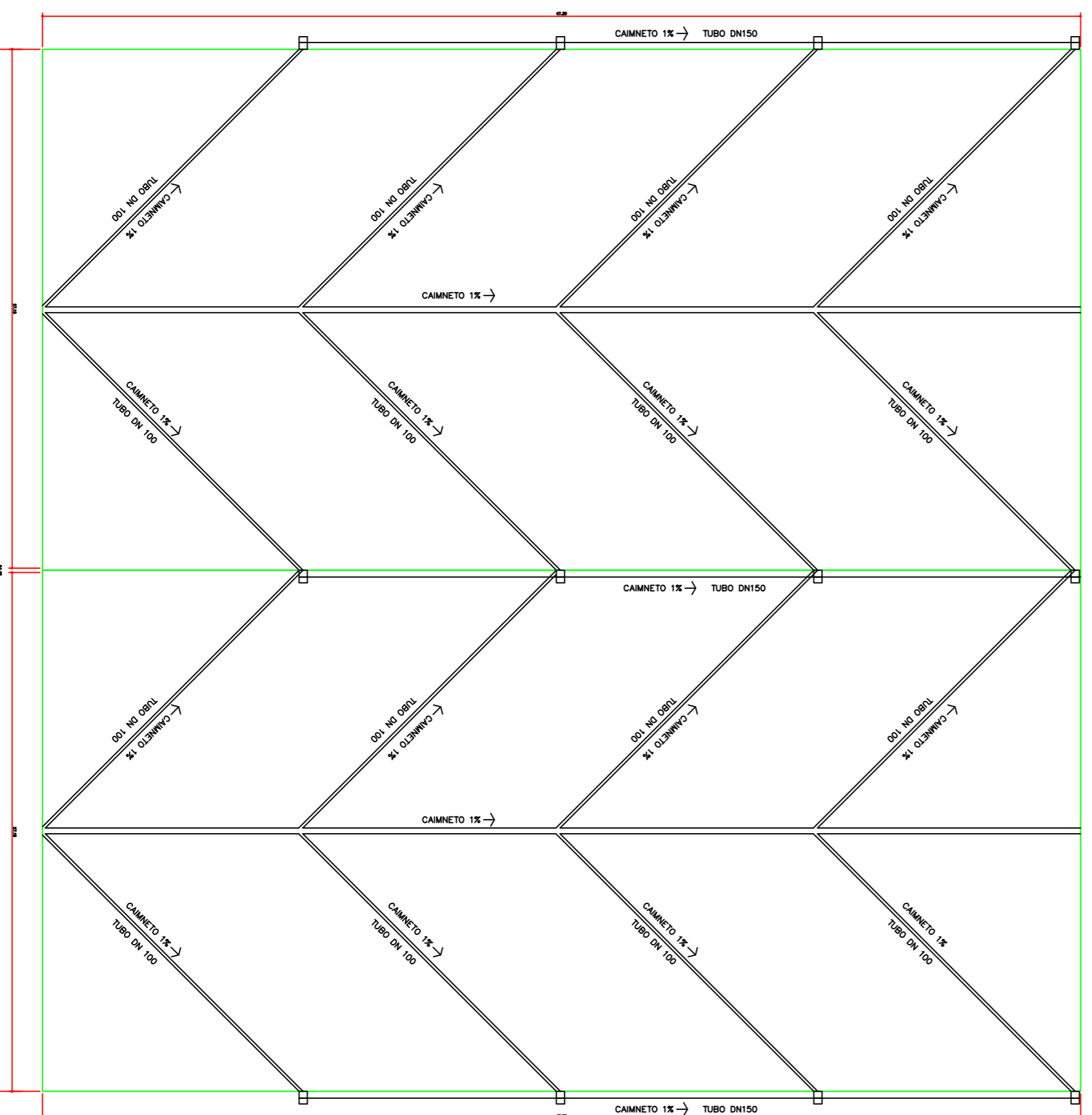
ESQUEMA DE DRENAGEM SUBTERRÂNEA ESPINHA DE PEIXE - FUTEBOL SOCIETY
