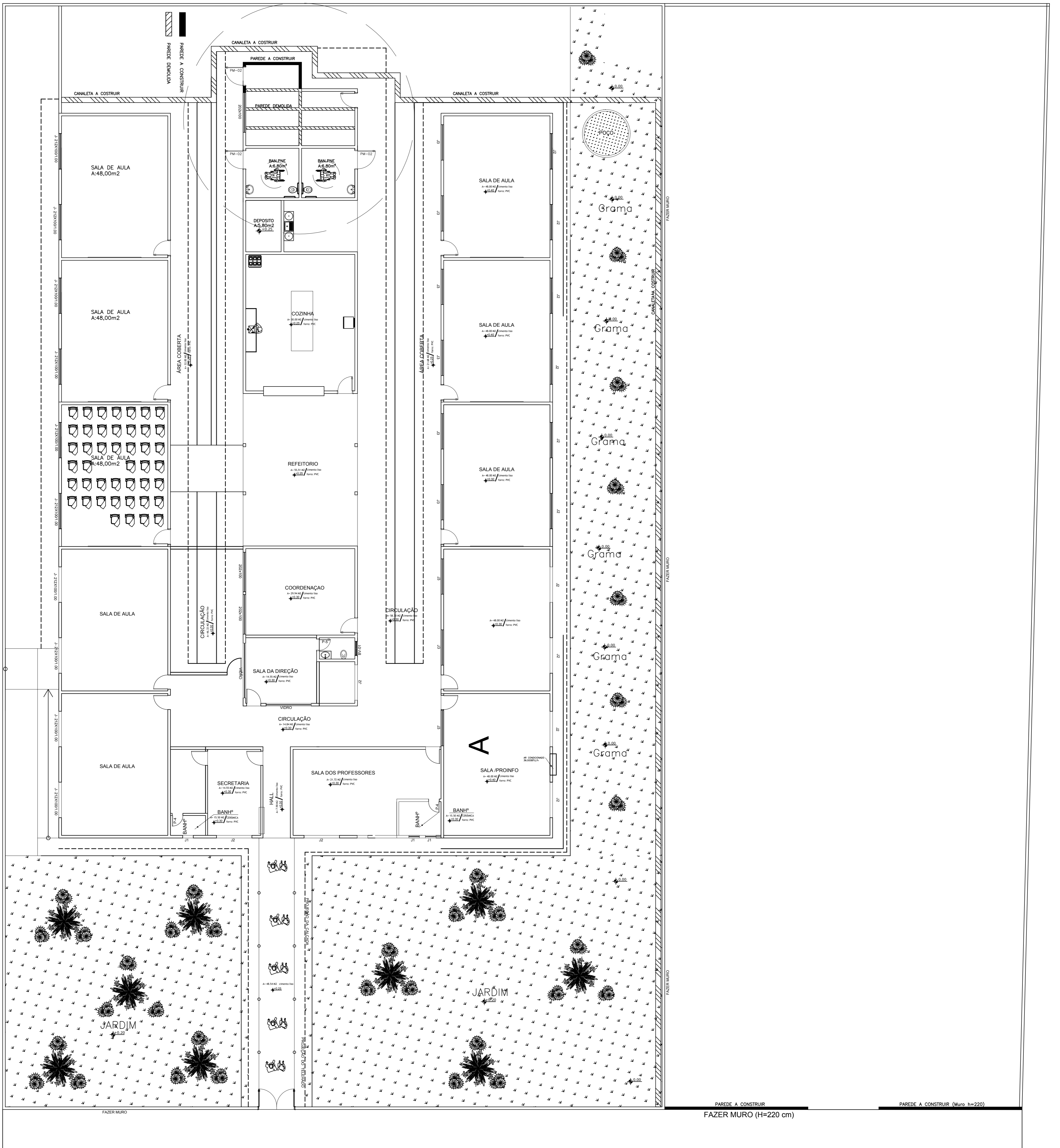
PLANTA BAIXA - PAVIMENTO TÉRREO ESCALA 1:50
