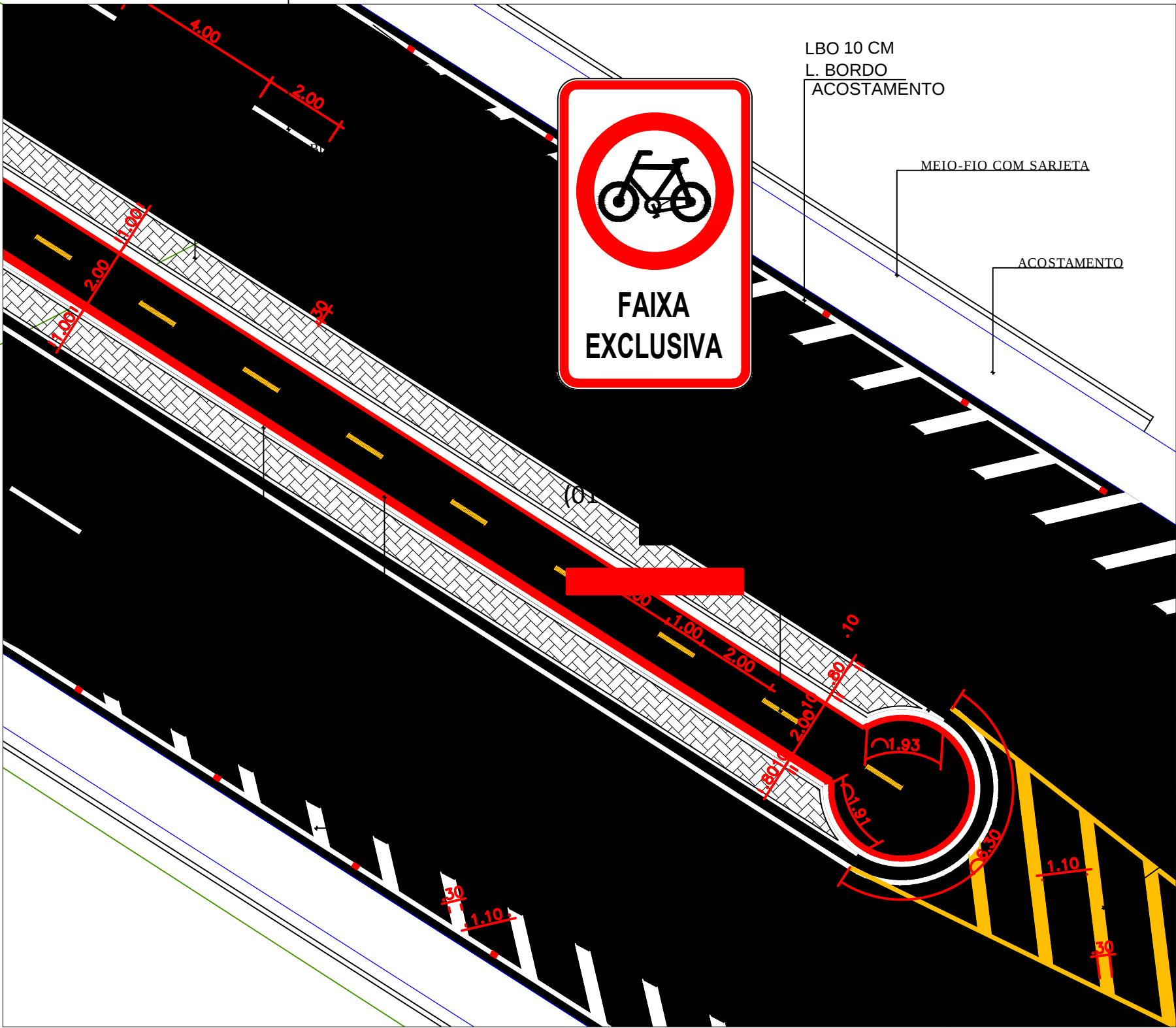
DETALHE A S/ESC.
