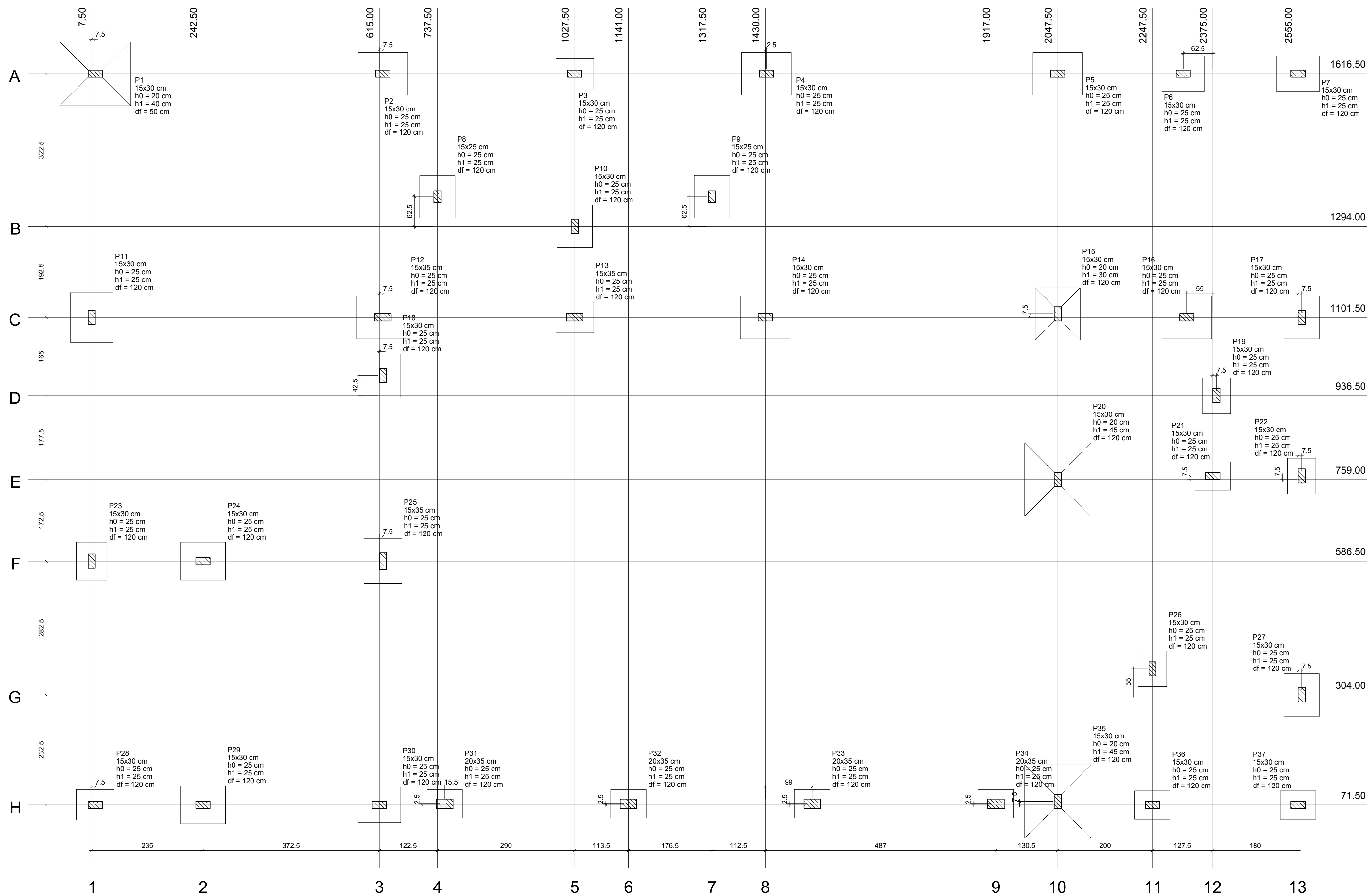
PLANTA DE LOCAÇÃO Escala 1:100
