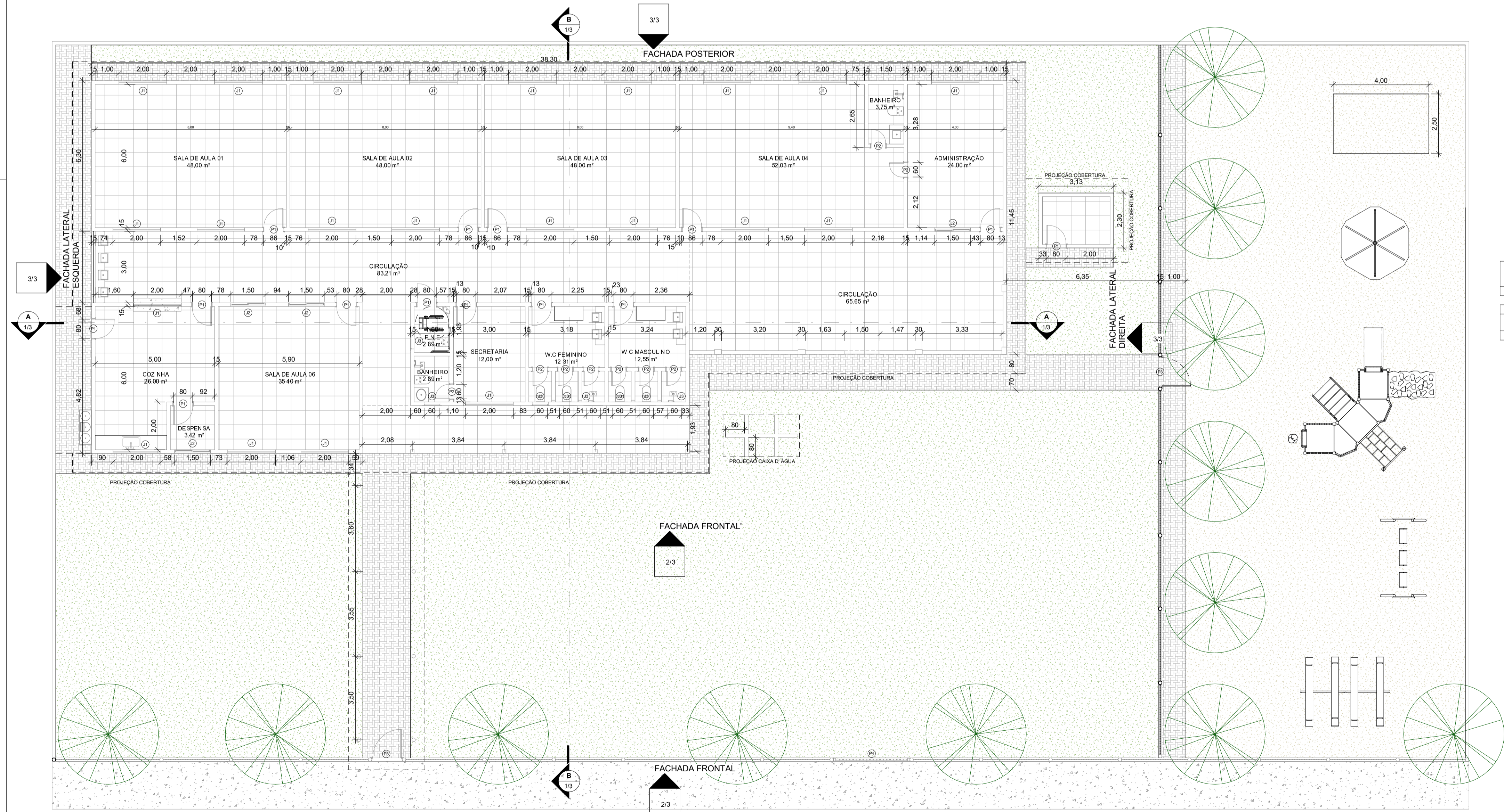
1 TÉRREO REFORMA 1 : 100
